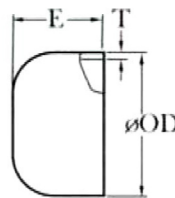
管帽 Cap
