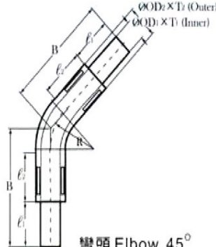
彎頭 Elbow 45°
