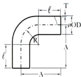
彎頭 90° Elbow
