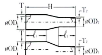
大小頭 Reducer
