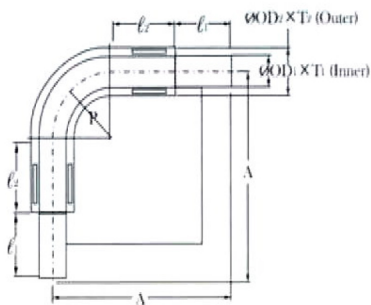
彎頭 Elbow 90°
