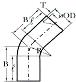
彎頭 45° Elbow
